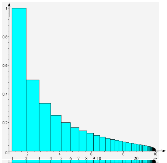
Рис. 4: Фінітизоване зображення гармонічного ряду
